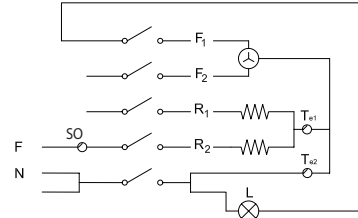
Manuel Kontrol Üniteli Fanlı Isıtıcı Elektrik Devre Şeması
