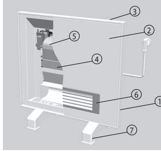
Elektrikli Manuel Fanlı Isıtıcı
